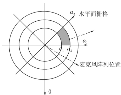
图 16 平面栅格
