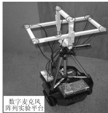
图3 8通道麦克风阵列
