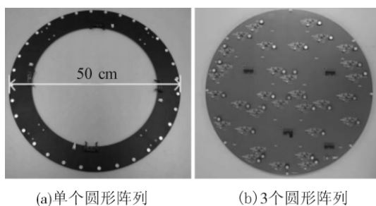
图 5 32 通道二维麦克风阵列
